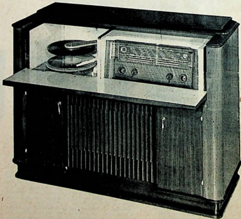
Twee concertluidsprekers in acoustische box als typische inslag van de Philips radiogramfoon FX 804 A. Basis van dit salonapparaat is een 15-buizen AM/FM chassis met balansuitgang
