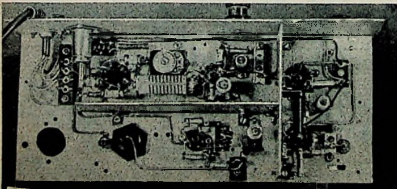
Interne uitvoering van de booster
