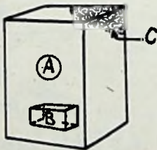
Fig. 2. Basreflexkast, waarin de luidspreker A en de pijp B, waardoor de tegen de achterwand gereflecteerde lage tonen kunnen uittreden. C is de geluidabsorberende bekleding. Ruimtelijke omvang en afmeting van luchtspleet B staan in een bepaalde verhouding ten opzichte van het type luidspreker.
