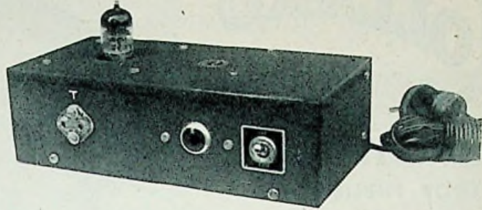
„Wisa“ antenneversterker
