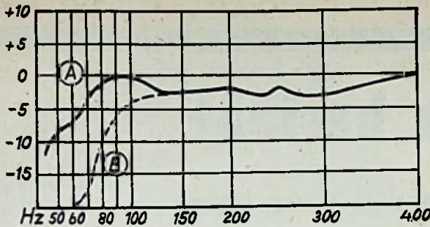
Fig. 1. Basweergave van goede luidspreker met groot klankscherm. In B de door gebruik van een te klein klankbord ontstane verzwakking.
