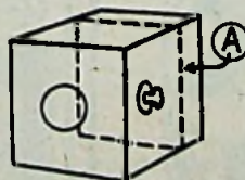
Fig. 3. Principe van de acoustische box. De kast is een kubus van ca. 50 x 50 x 50 cm, wanden aan de binnenzijde bekleed. A is een viltplaat waarmee de kast wordt 'afgestemd' op het luidsprekersysteem.
